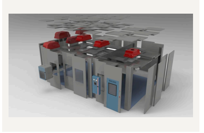
Konsept Modüler Temiz Oda
